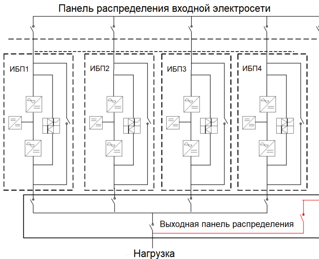
Рисунок 5.9. Схема параллельного подключения ИБП
