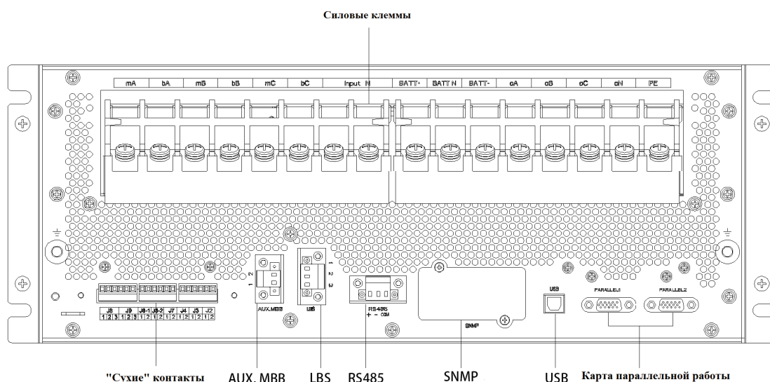
Рисунок 2.2-1. Вид задней панели ИБП 30-40 кВА
