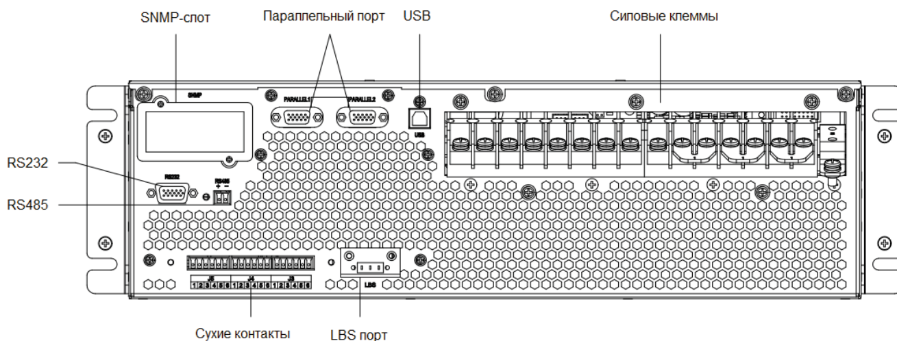
Рисунок 3.6. Коммуникационные интерфейсы
