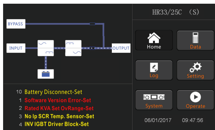
Рисунок 5.7. Запуск ИБП от батарей
