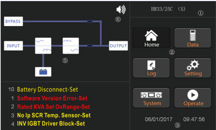
Рисунок 4.2. Домашняя страница
