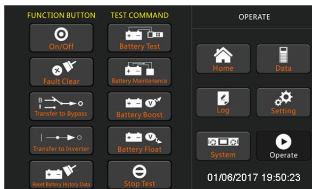
Рисунок 4.12. Меню управления
