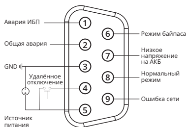
а. Разъём DB9
